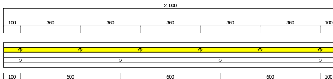
2000 L 正面図
