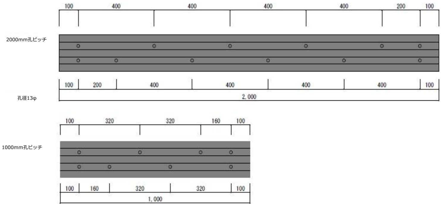
PCE-4012 PCE-6015NS PCE-6018 正面図
